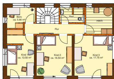
Grundriss OG
